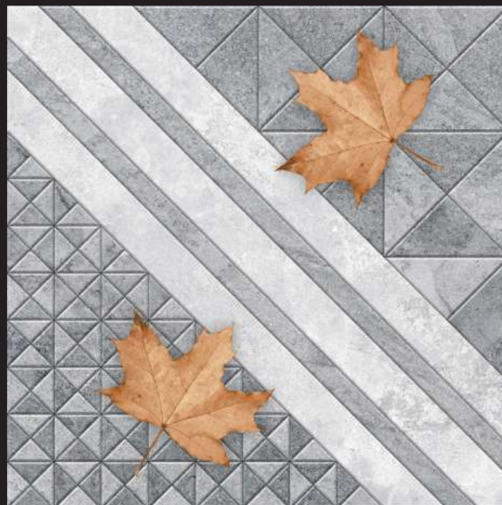
AGATE-115
